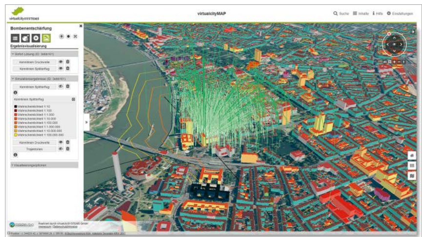
Abbildung 1: Virtuelle Simulation des berechneten Splitterfluges. Bild: Fraunhofer EMI
