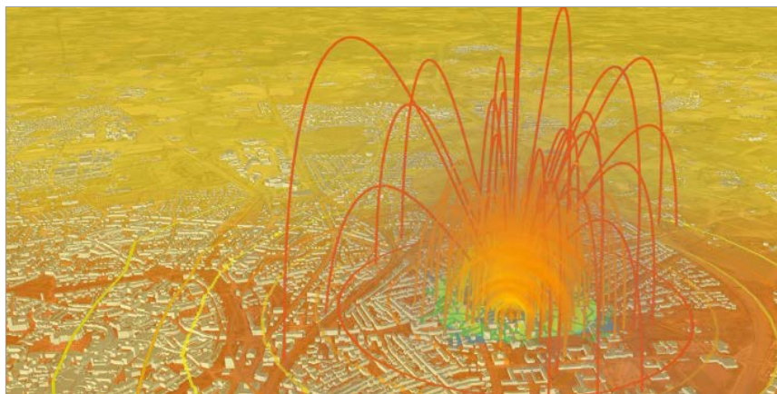
Abbildung 2: Basierend auf 3D-Stadtmodellen kann man die Druckwellenausbreitung und den Splitterflug bei einer Bombendetonation simulieren. Bild: Fraunhofer EMI
